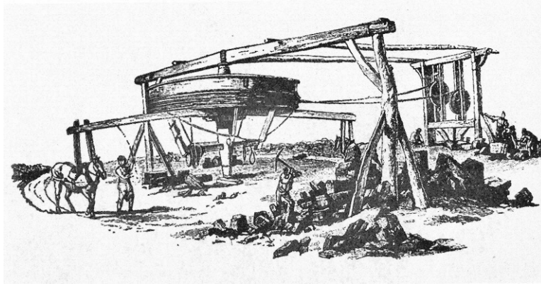
Kezdetleges gépesített külszíni fejtés; Anglia; XVIII. század
